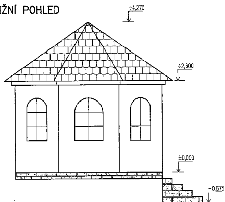
JIŽNÍ POHLED
